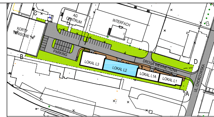
ORIENTACJA 1:250
